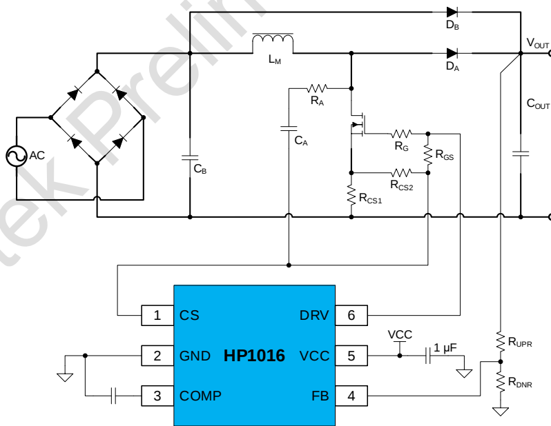
Figure 1 典型应用电路
