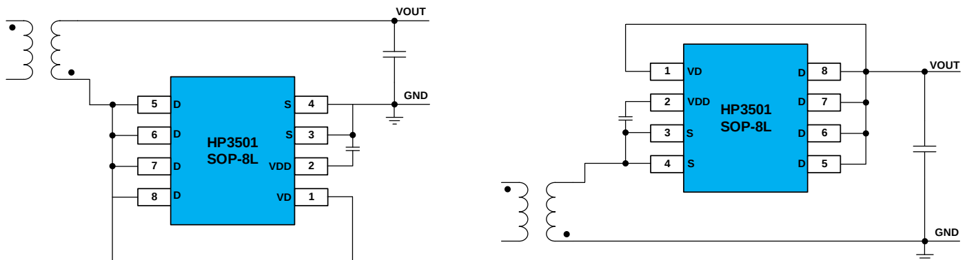
图 1. 典型应用电路
